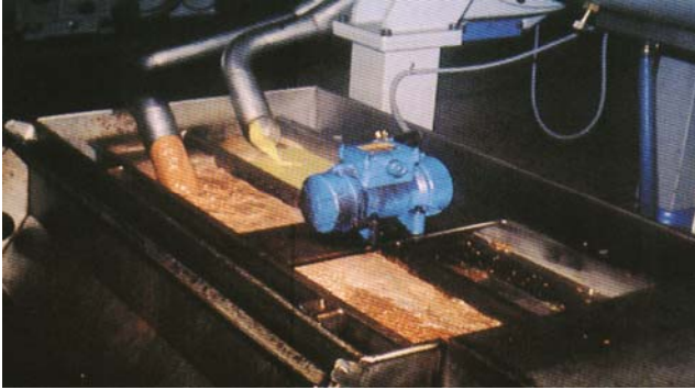
Figura 15.- Tamiz vibratorio en la salida de los líquidos del decantador centrífugo
