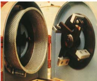
Figura 11.- Interior de un molino de martillos
