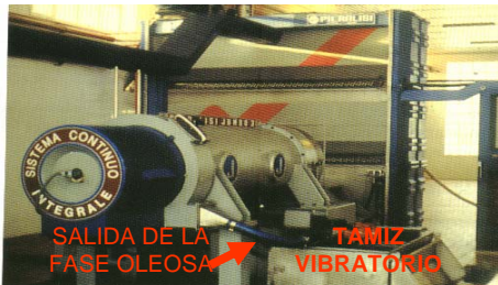
Figura 20.- Decantador de dos fases
